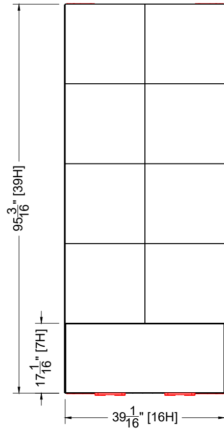
FRONT ELEVATION Scale: 1/2" = 1'-0"
